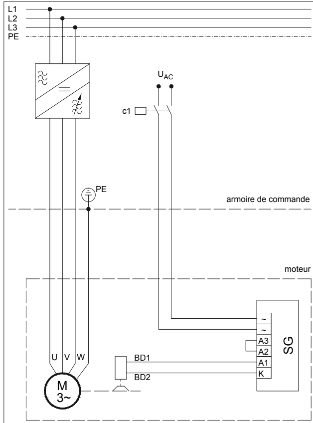
Figure 7: Alimentation séparée du redresseur.
