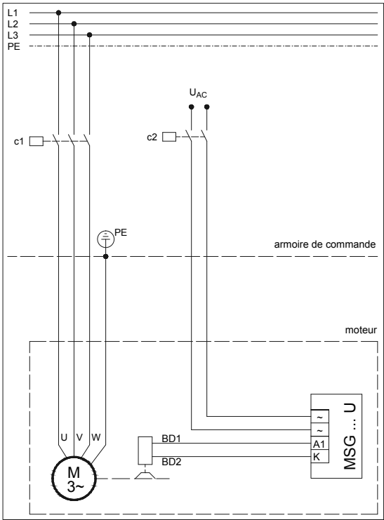
Figure 9: Alimentation frein: Redresseur standard
