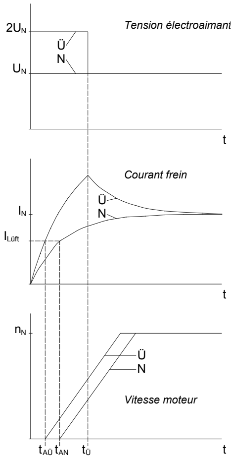
Figure 2: Schéma de principe de la tension de la bobine, du courant de la bobine et de la vitesse de rotation du moteur en excitation normale (N) et en surexcitation ( \ddot{U} ).
