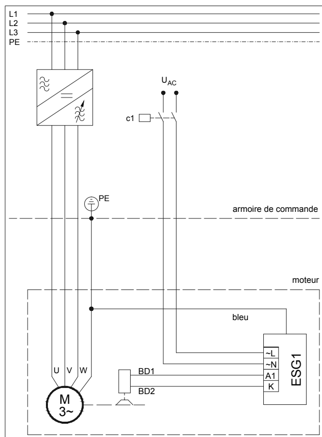
Fig.8a: Alimentation séparée du redresseur par ex. en cas d'alimentation par variateur
