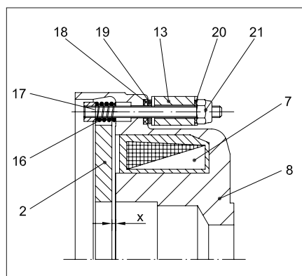
Figure 12: Montage du dispositif de desserrage manuel
