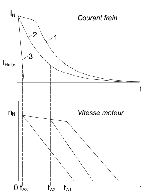
Figure 3: Evolution de principe du courant de la bobine et de la vitesse de rotation du moteur après coupure du circuit à courant alternatif (1, 2) et du circuit à courant continu (3)
