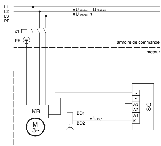
Figure 5: Coupure du circuit à courant alternatif → Bornes A2 et A3 pontées
