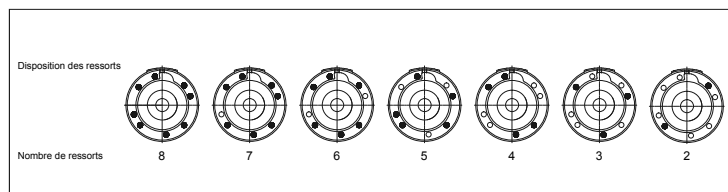
Figure 14: Disposition des ressorts en cas de réduction de couple
