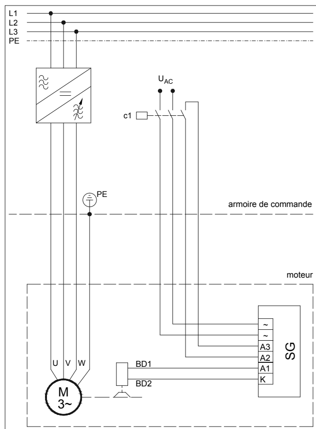
Fig.7a: Alimentation séparée du frein. Coupure du circuit continu par contact aux bornes A2 et A3.
