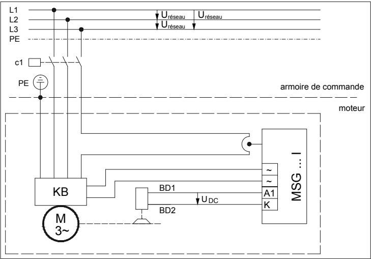
Figure 10: Alimentation du redresseur provenant du bornier moteur KB (voir raccordement du redresseur au moteur KB)
