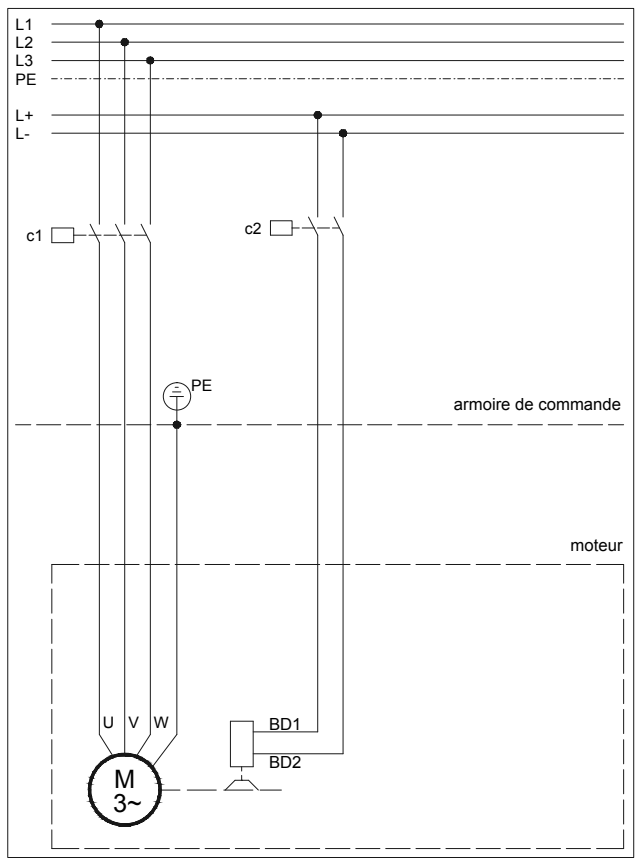
Figure 4: Alimentation directe en tension continue à partir d'un circuit de commande
