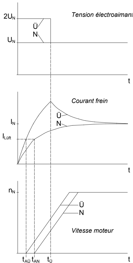
Figure 2: Schéma de principe de la tension de la bobine, du courant de la bobine et de la vitesse de rotation du moteur en excitation normale (N) et en surexcitation (S).
