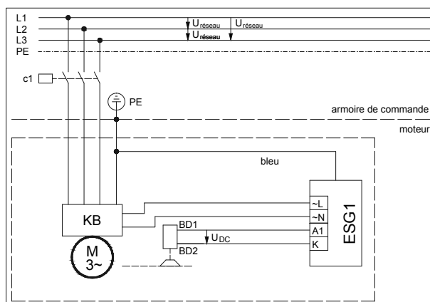
Figure 8: Alimentation du redresseur à partir de la plaque à bornes du moteur Alimentation du redresseur provenant du bornier moteur KB (voir raccordement du redresseur au moteur KB)
