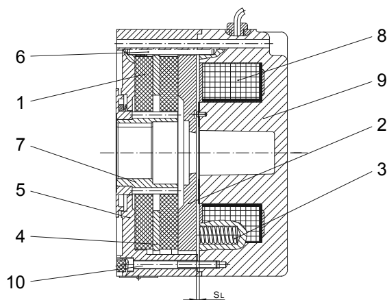
Figure 1: Freins à ressort à deux disques de la série Z..
