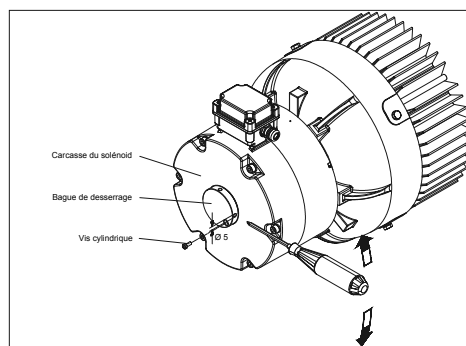
Figure 12: Frein de types E../Z..075 et Z..100 - avec desserrage manuel verrouillable
