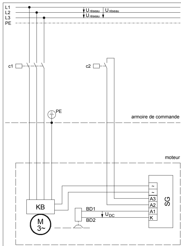
Figure 6 : Coupure du circuit à courant continu aux bornes A2 et A3 par ex. par un contact de contacteur.
