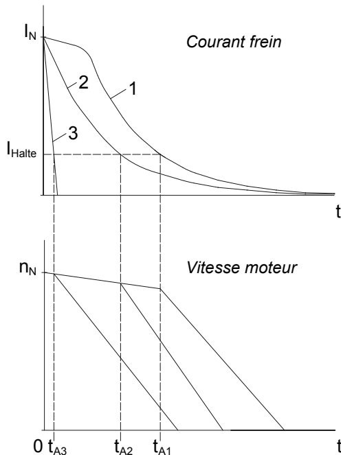
Figure 3: Evolution du courant de la bobine et de la vitesse de rotation du moteur après coupure du circuit à courant alternatif (1, 2) et du circuit à courant continu (3).
