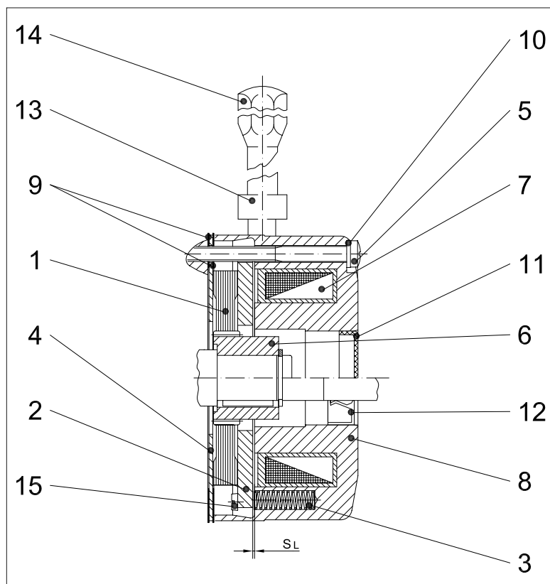
Figure 1: Frein à ressort de la série E003B ou E004B
